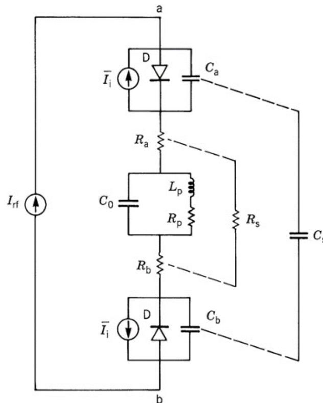
Slika 1.1.7 Model ekvivalentnog električnog kola kojim se opisuju nelinearne električne osobine homogenog radiofrekventnog pražnjenja [6]
