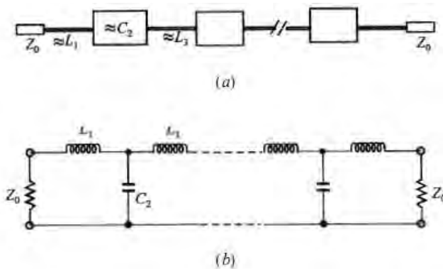
Slika 1. (a) Aproximirani model NF filtra sa vodovima, (b) LC šema NF filtra sa vodovima.
