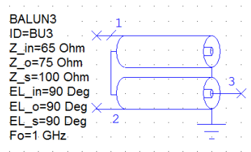
Слика 2. Маршанов балун у AWR-у.
