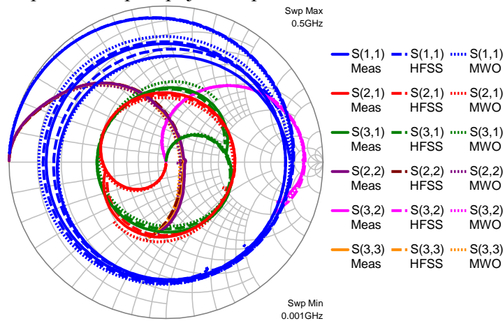
Слика 8. Резултати симулација у АWR-у, HFSS-у и резултати мерења на лабораторијском прототипу.
