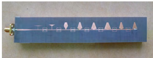
Sl. 6. Izgled realizovanoog antenskog niza sa pentagonalnim dipolima i kontinualnim prelazom sa balansnog na nebalansni vod na ulazu.
