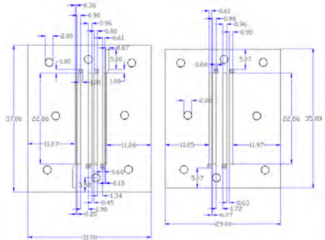
Слика 2. Плочице филтера са димензијама у mm.
