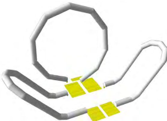
Слика 7. Тродимензионални приказ модела балуна у АWR-у.
