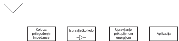
Sl. 1. Elementi sistema za prikupljanje i konverziju RF energije.
