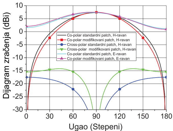
Sl. 7. Dijagrami zračenja modificovanog peča i standardnog na 17 GHz.
