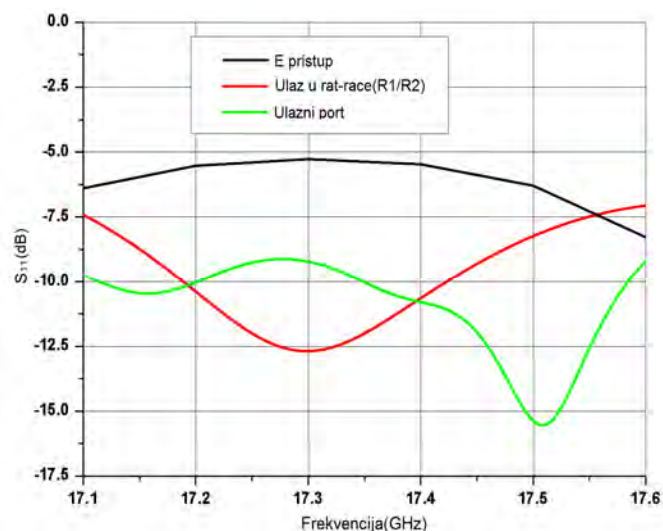
Sl. 5. S_{11} -parametar na različitim mestima napojne mreže na Sl. 4.
