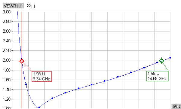
Slika 5a. VSWR za spregnute Bow-tie na 100 oma.
