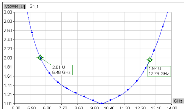
Slika 5c. VSWR za spregnute petougaone dipole na 100 oma.
