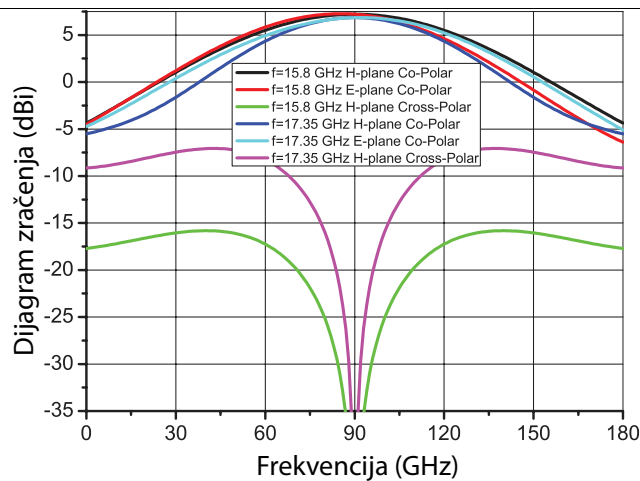
Сл. 4. Дијаграм зрачења на у обе равни на првој и другој резонанси.
