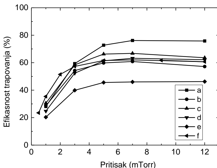
Slika 5.11 Efikasnost predloženog dizajna trapa u funkciji pritiska CF_4 u prvom stepenu za različite modele diferencijalnog preseka za elastično rasejanje pozitrona na CF_4 . Oznake u legendi odgovaraju modelima diferencijalnog preseka prikazanim na slici 5.10.
