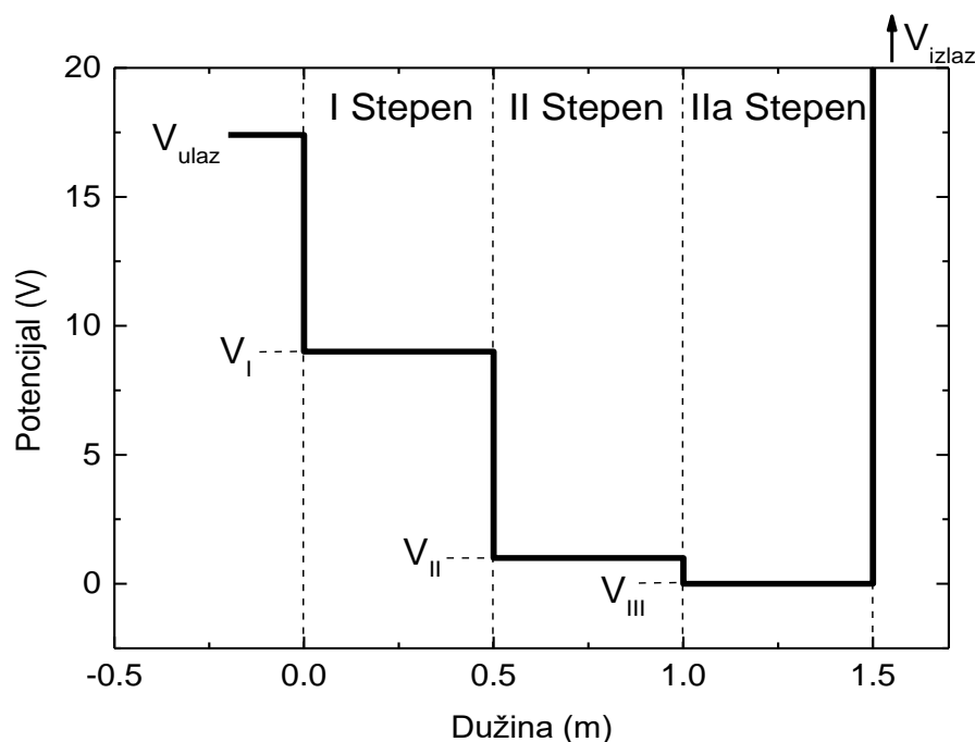
Slika 4.16 Profil električnog potencijala na elektrodama u modelu dvostepenog pozitronskog trapa.
