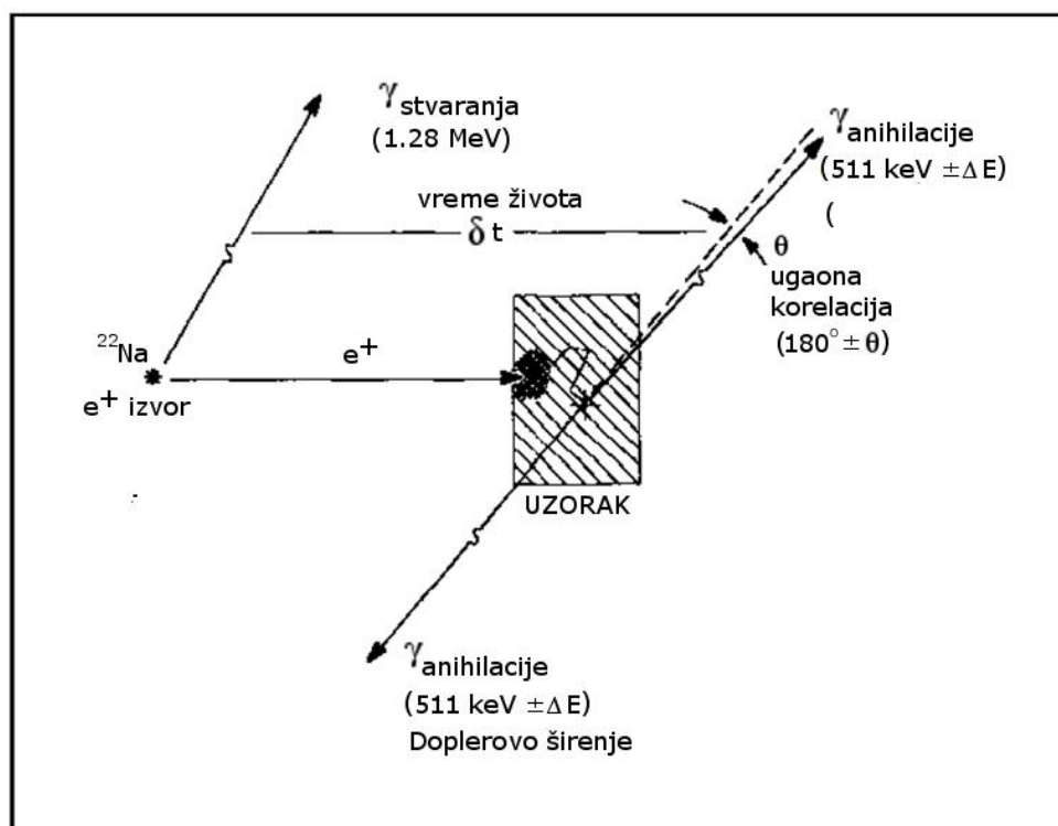
Slika 1.9 Šematski prikaz anihilacije pozitrona koji prikazuje osnove tri tehnike koje se koriste u pozitronskoj anihilacionoj spektroskopiji: merenje vremena života, ugaone korelacije i Doplerevog širenje. (Siegel, 1980)
