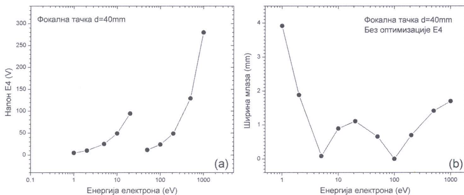
СЛИКА 2. а) Зависност напона E4 од енергије, тако оптимизованог да се увек добије фокално растојање d=40\text{mm} . б) Зависност ширине електронског млаза од енергије на фокалном растојању d=40\text{mm} од последње електроде електронског топа, без оптимизације напона на електроди E4.
